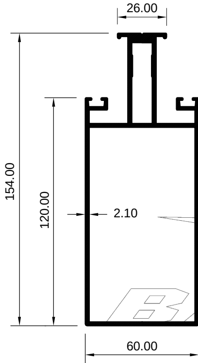
ART 3029344 (KG/MTR = 2.918)
