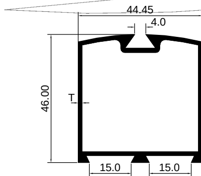
DOOR VERTICAL
