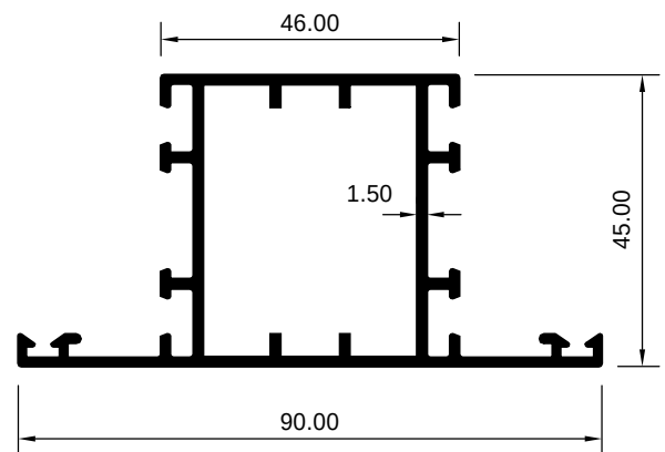
ART 2008063 (KG/MTR = 1.176)
