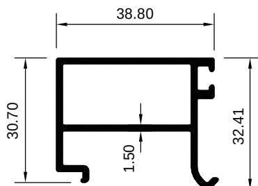
ART 1029298 (KG/MTR = 0.606)
