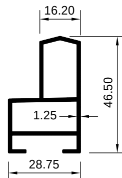
ART 2029098 (KG/MTR = 0.563)
