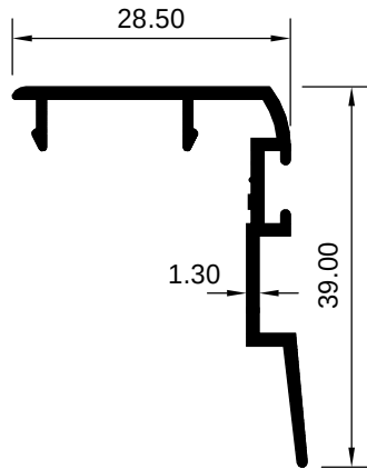
ART 1007871 (KG/MTR = 0.293)
