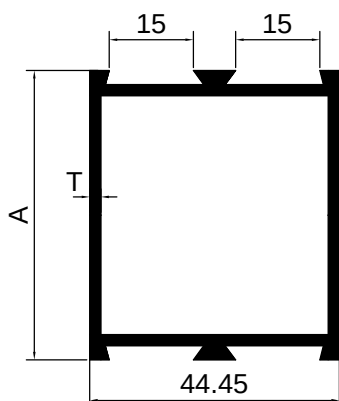
DOOR MIDDLE
