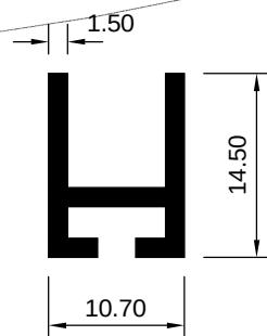
ART 1007804 (KG/MTR = 0.167)
