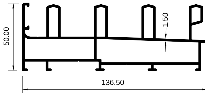
ART 3008006 (KG/MTR = 2.459)
