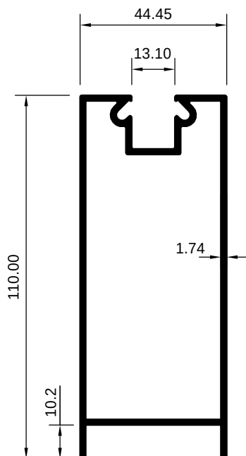
ART 2029024 (KG/MTR = 1.627)
