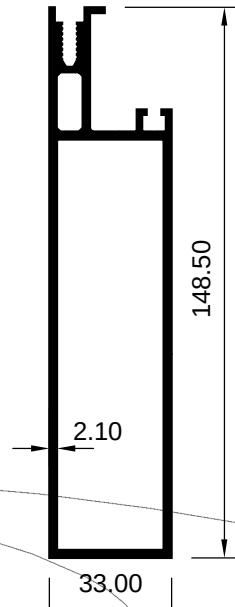
ART 3008057 (KG/MTR = 2.181)
