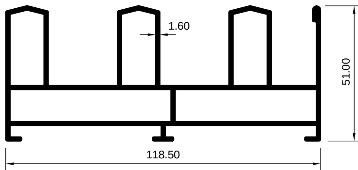
ART 2029292 (KG/MTR = 2.370)
