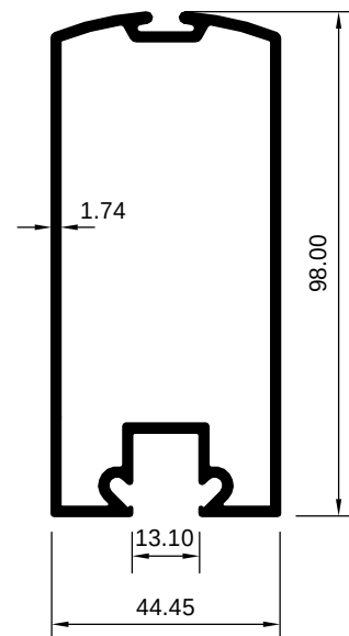
ART 2029027 (KG/MTR = 1.545)
