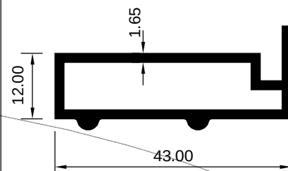
ART 2007809 (KG/MTR = 1.628)
