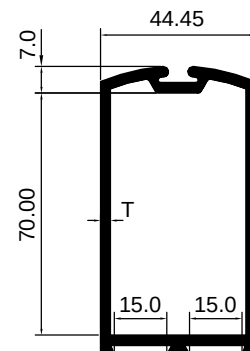
DOOR VERTICAL
