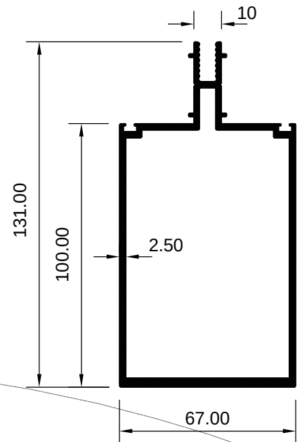
ART 2008035 (KG/MTR = 1.570)
