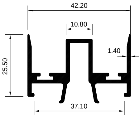
ART 1029269 (KG/MTR = 0.646)
