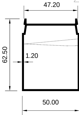
ART 1029172 (KG/MTR = 0.723)
