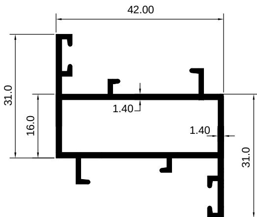
ART 1005581 (KG/MTR = 0.618)
