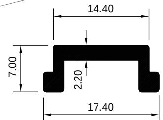
ART 1029325 (KG/MTR = 0.147)
