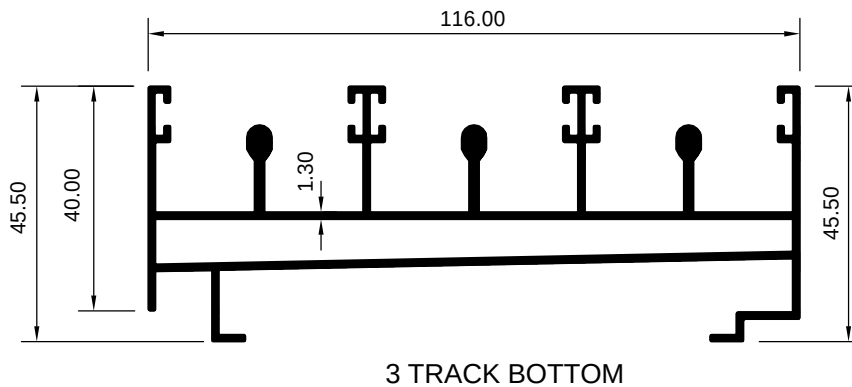
ART 2029041 (KG/MTR = 1.854)
