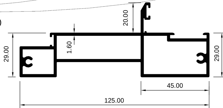
ART 3029076 (KG/MTR = 1.807)
