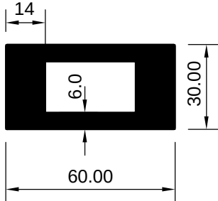
ART 3029090 (KG/MTR = 3.304)
