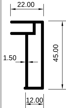
ART 2008084 (KG/MTR = 0.541)
