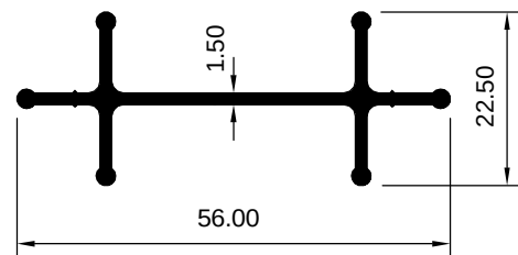
ART 2007811 (KG/MTR = 0.539)
