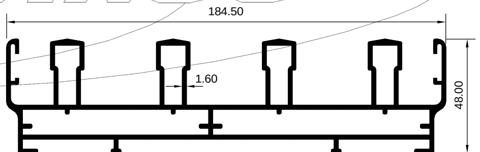
ART 3029353 (KG/MTR = 3.502)
