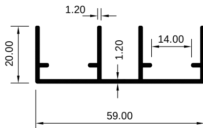
ART 1029047 (KG/MTR = 0.475)
