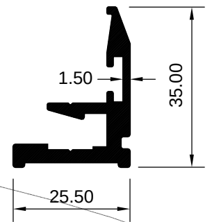
ART 2029073 (KG/MTR = 0.600)
