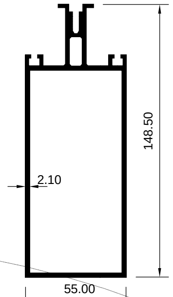
ART 3008056 (KG/MTR = 2.500)
