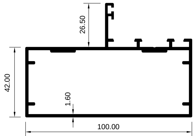
ART 2029216 (KG/MTR = 1.626)
