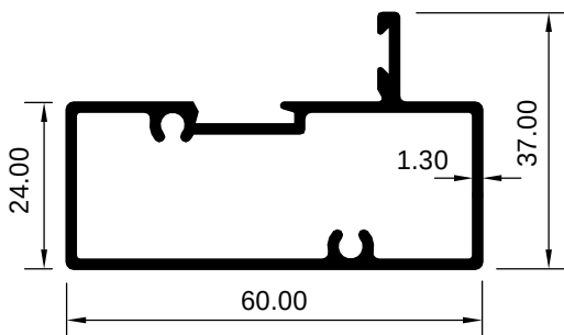
ART 1029232 (KG/MTR = 0.732)
