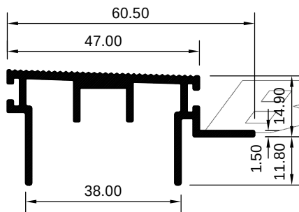
ART 1029273 (KG/MTR = 0.700)
