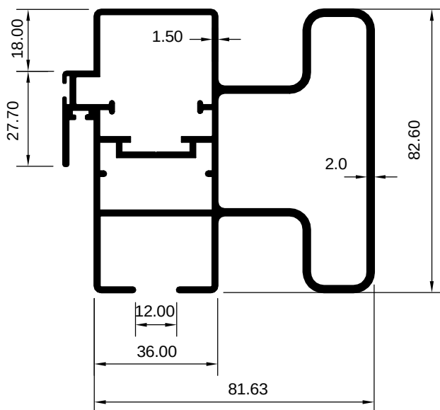
ART 3008062 (KG/MTR = 2.563)
