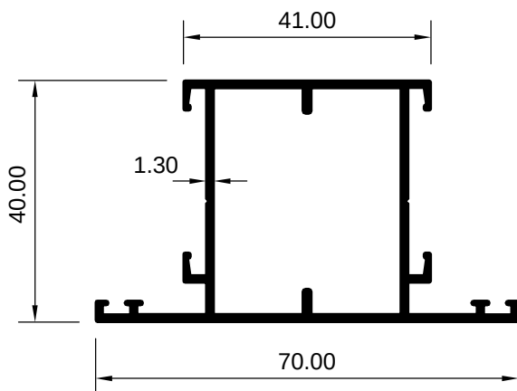
ART 1007999 (KG/MTR = 0.789)
