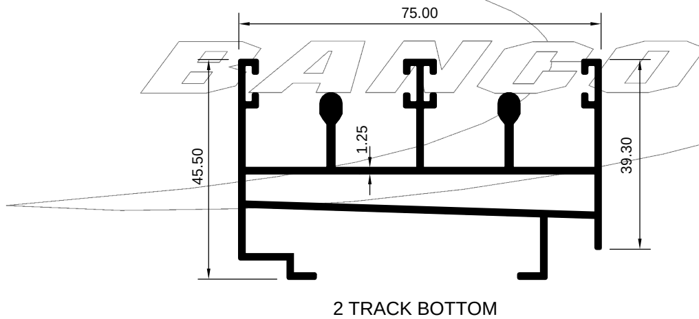
ART 2029039 (KG/MTR = 1.286)
