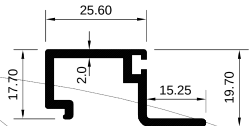
ART 1029356 (KG/MTR = 0.441)
