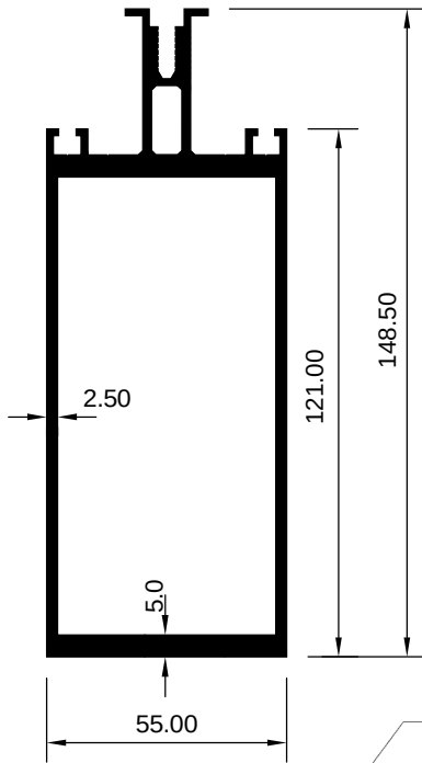
ART 3007826 (KG/MTR = 3.533)
