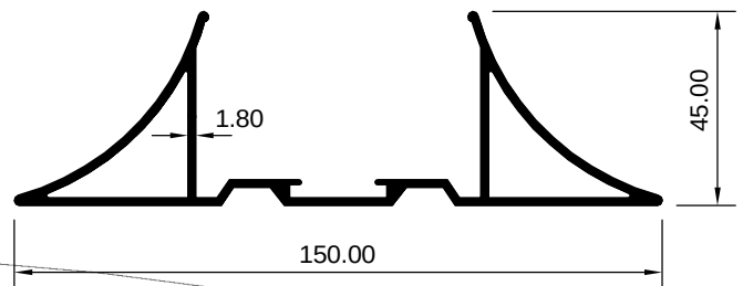
ART 3007814 (KG/MTR = 1.771)
