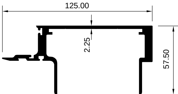
ART 3008034 (KG/MTR = 2.116)
