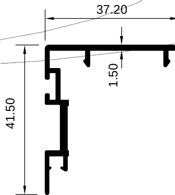
ART 2029292 (KG/MTR = 2.370)
