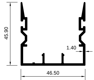
ART 1029268 (KG/MTR = 0.686)
