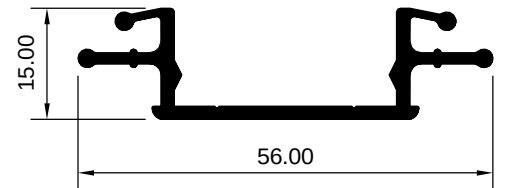
ART 3007814 (KG/MTR = 1.771)
