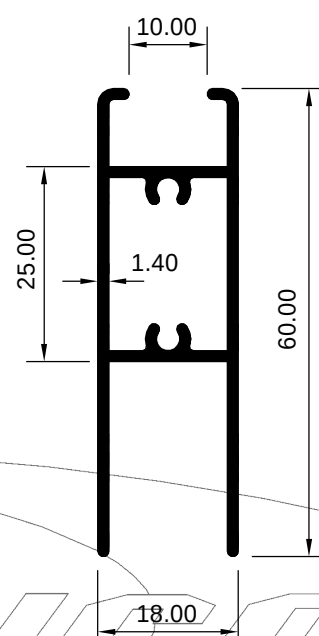
ART 1007841 (KG/MTR = 0.637)
