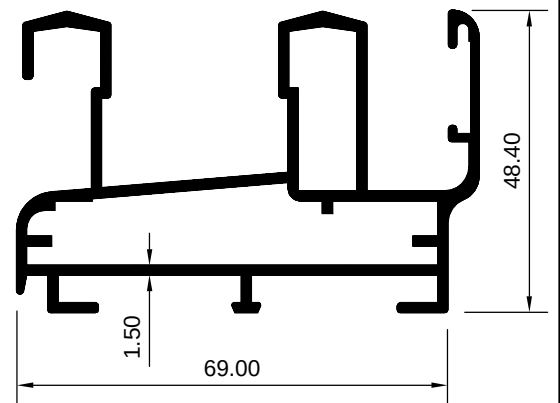
ART 2008054 (KG/MTR = 1.489)
