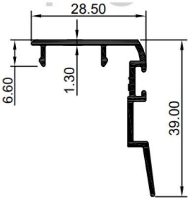
INTERLOCK
