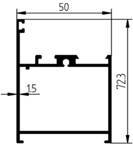
DOOR BOX FRAME
